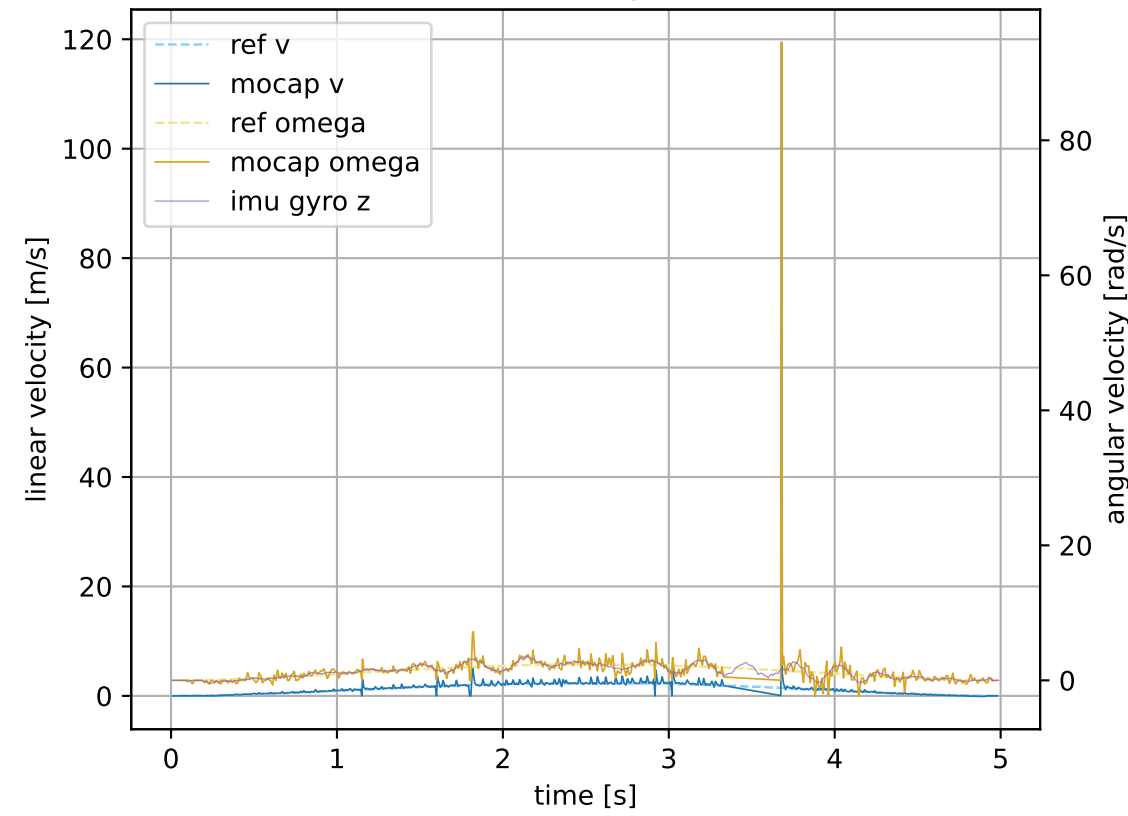
y State
